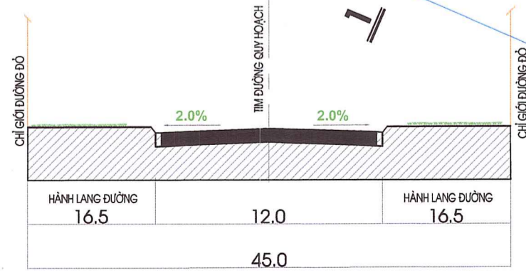
MẶT CẮT 2-2 (ĐƯỜNG TRÁNH QL38B)
