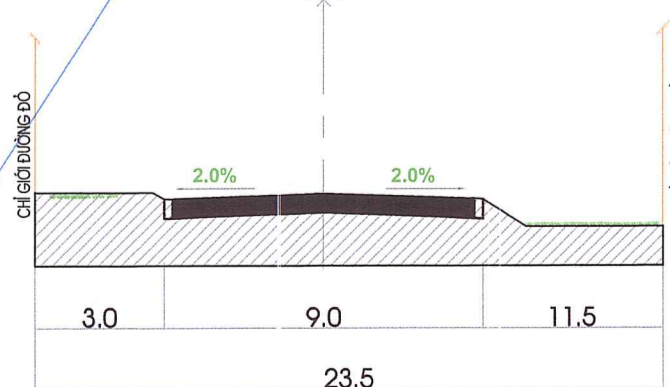
MẶT CẮT 1-1 (ĐƯỜNG HUYỆN 20C)
