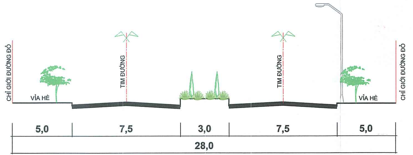
MẶT CẮT 1-1 (ĐƯỜNG NỘI BỘ CỤM CÔNG NGHIỆP)
