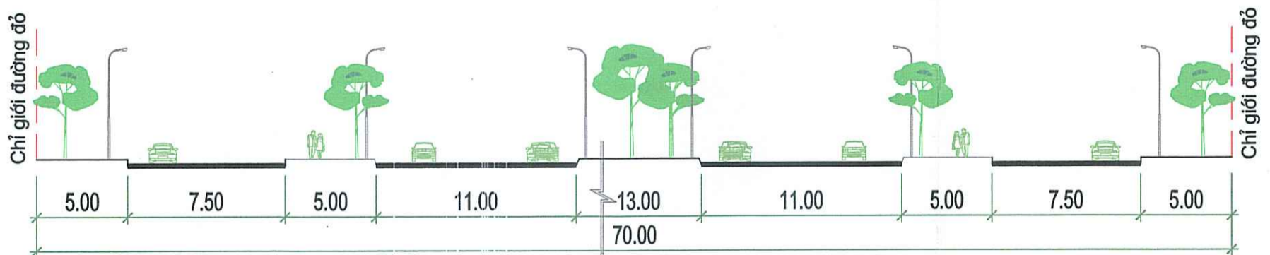
MẶT CẮT 4-4 (ĐƯỜNG 396)
