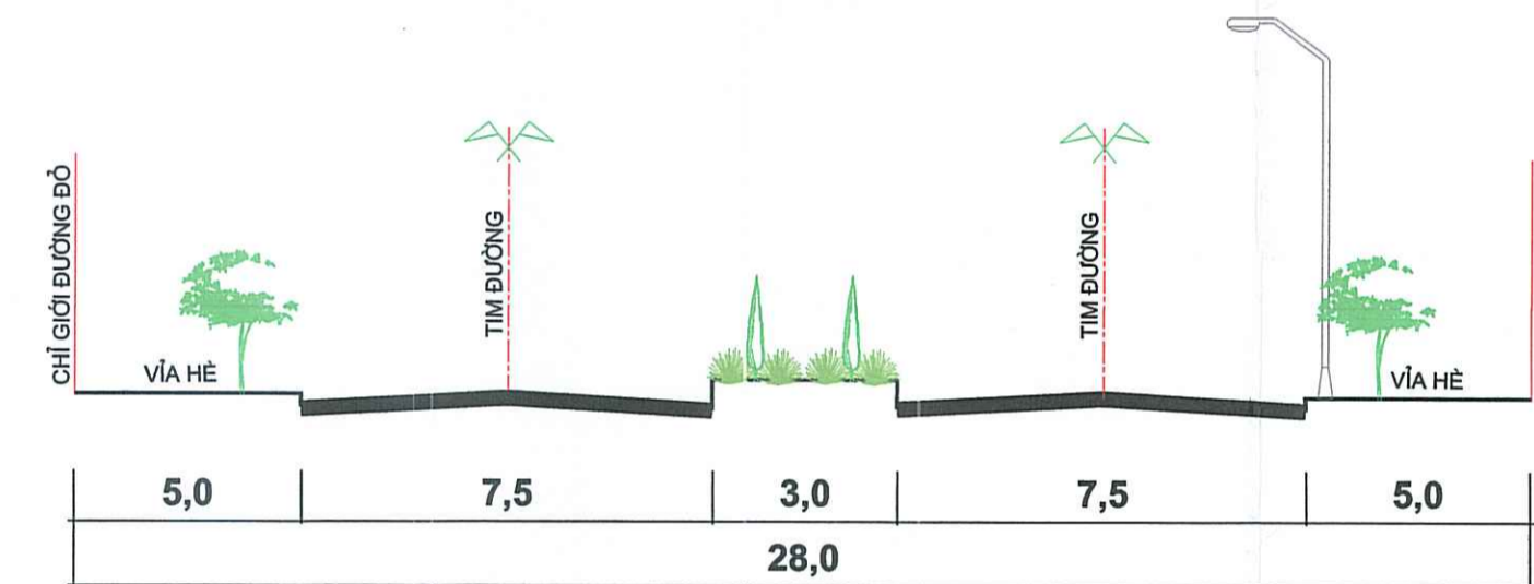
MẶT CẮT 1-1 (ĐƯỜNG NỘI BỘ CỤM CÔNG NGHIỆP)
