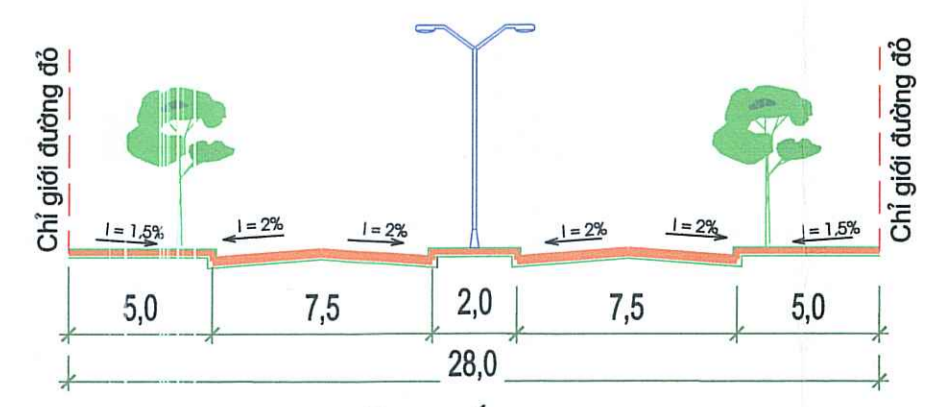
MẶT CẮT 2-2
