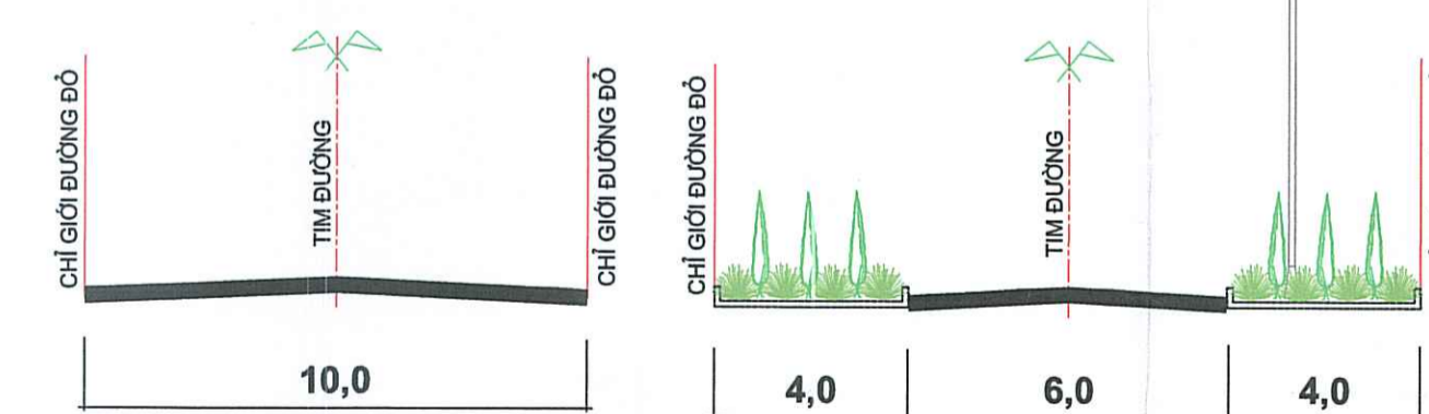
MẶT CẮT 3-3
