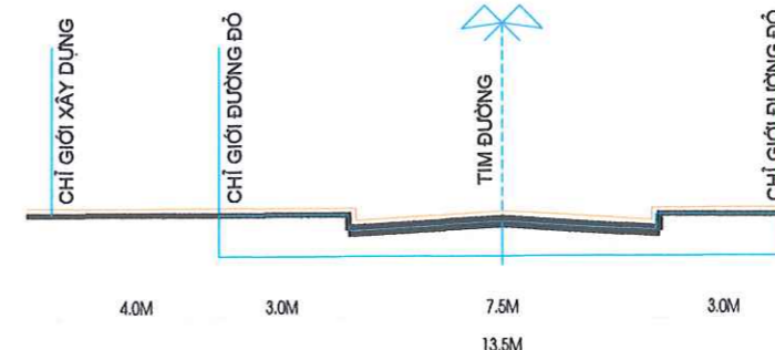
MẶT CẮT 1-1
