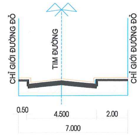
MẶT CẮT 2-2
