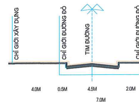
MẶT CẮT 2-2
