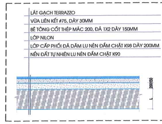
MẶT CẮT SÀN, ĐƯỜNG ĐIỂN HÌNH
