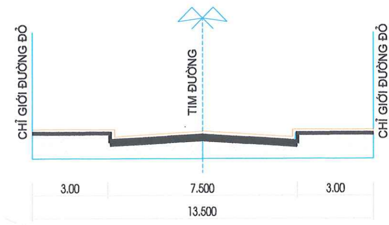
MẶT CẮT 1-1
