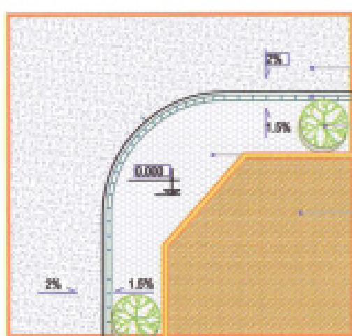
CT1 - CHI TIẾT MINH HỌA LỘ GIỚI KHU NHÀ LIỀN KỀ GÓC GIAO LỘ
