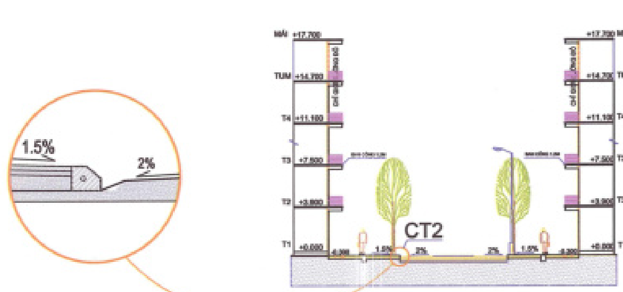
CT2 - MINH HỌA CHI TIẾT BỐ VÍA VÀ BÀNH THOÁT NƯỚC MẶT ĐƯỜNG
