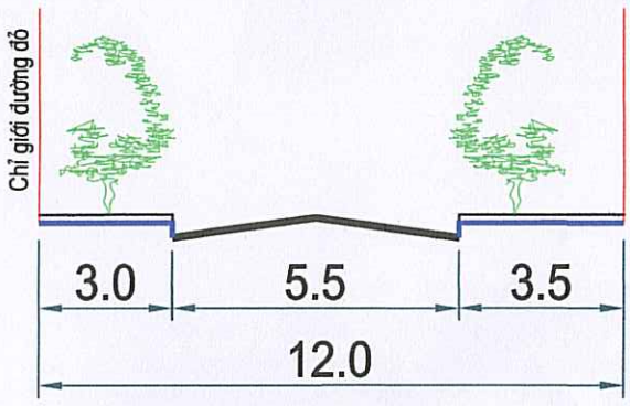
MẶT CẮT 4 - 4
