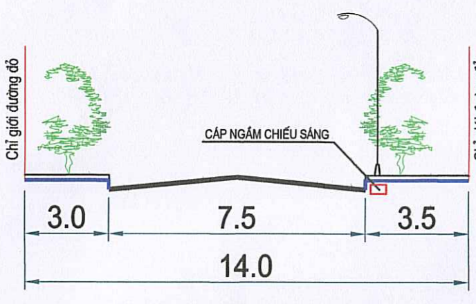
MẶT CẮT 3-3
