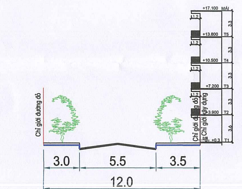
MẶT CẮT 4 - 4
