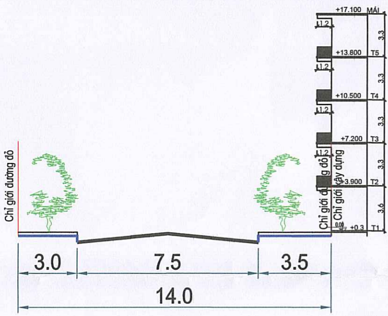
MẶT CẮT 3 - 3
