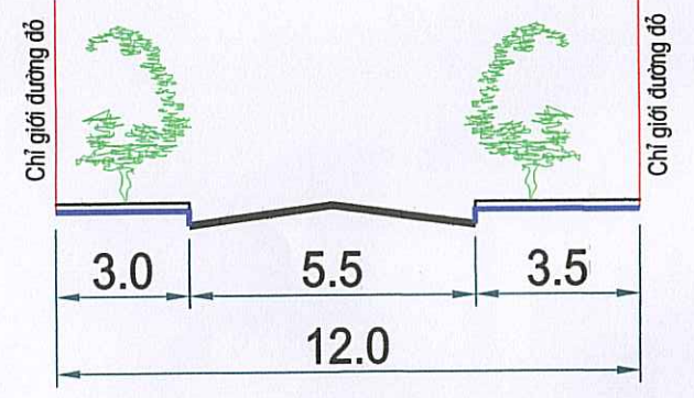
MẶT CẮT 4-4
