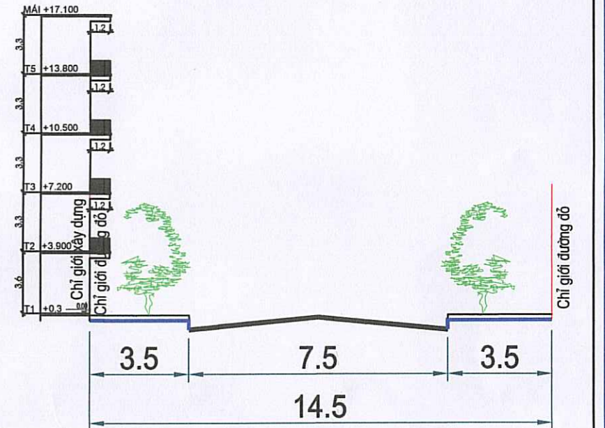
MẶT CẮT 2* - 2*
