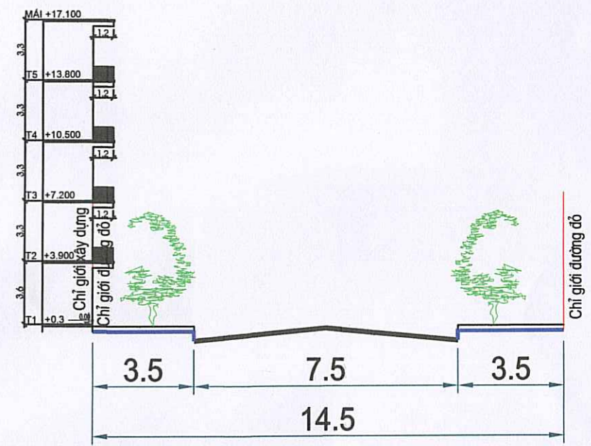
MẶT CẮT 2* - 2*
