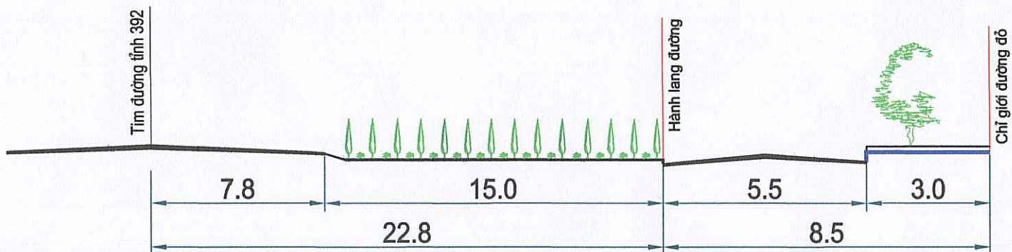
MẶT CẮT 1 - 1
