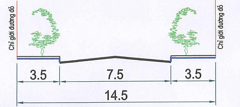
MẶT CẮT 2* - 2*
