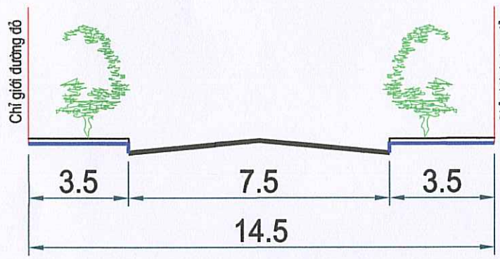
MẶT CẮT 2 - 2
