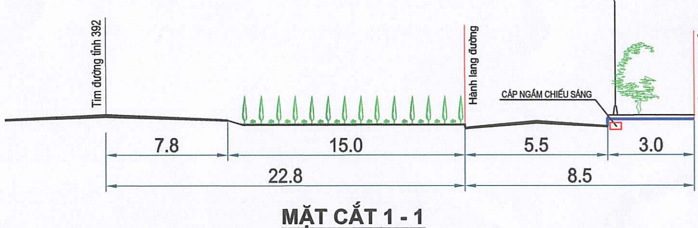
MẶT CẮT 1-1
