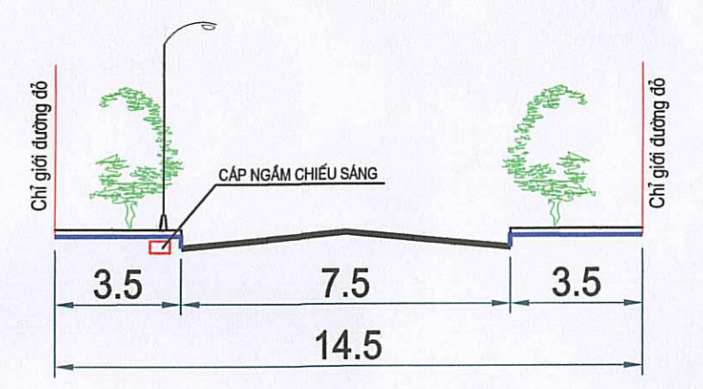
MẶT CẮT 2* - 2*
