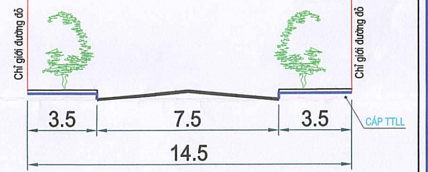
MẶT CẮT 2* - 2*
