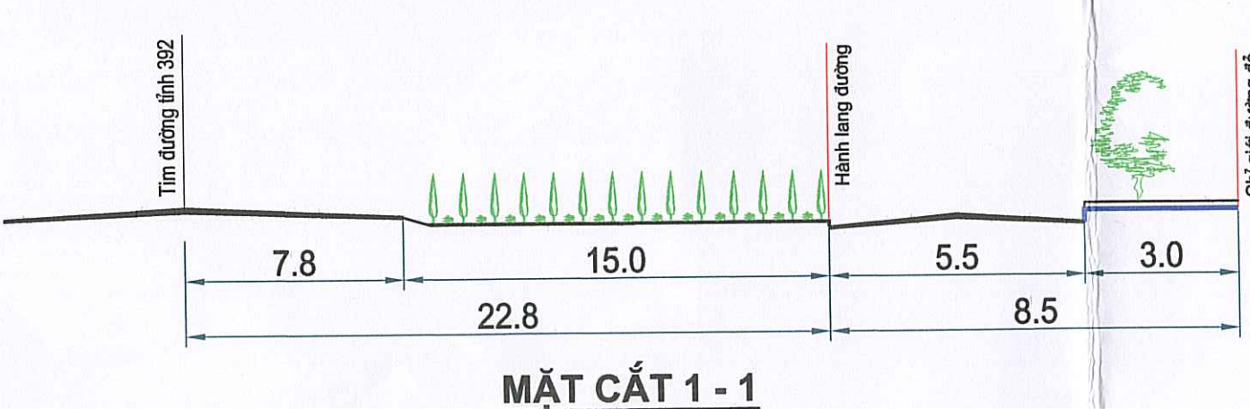
MẶT CẮT 1-1
