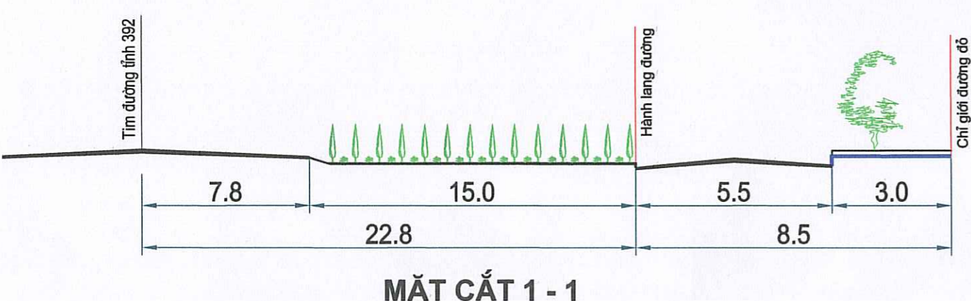
MẶT CẮT 1 - 1
