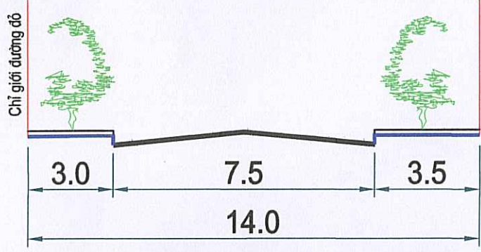
MẶT CẮT 3 - 3
