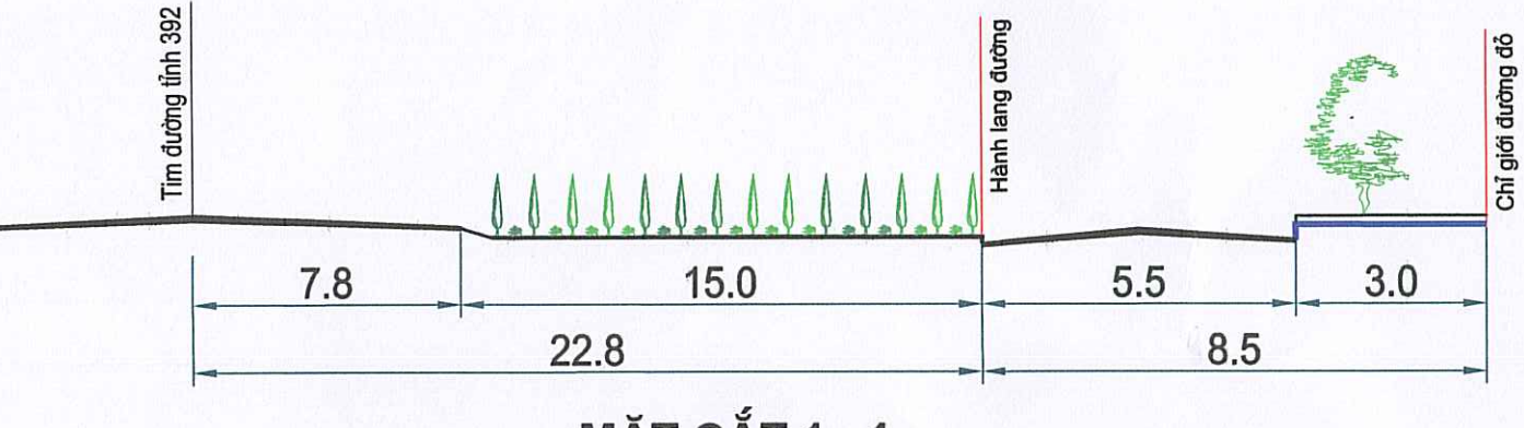
MẶT CẮT 1-1
