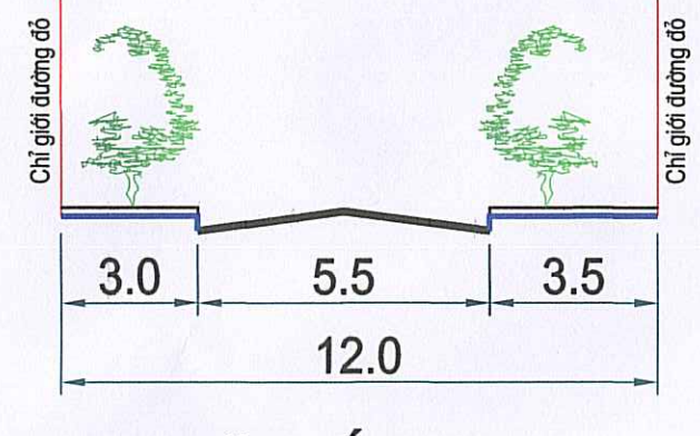
MẶT CẮT 4-4
