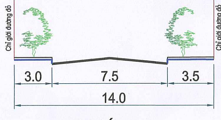
MẶT CẮT 3-3
