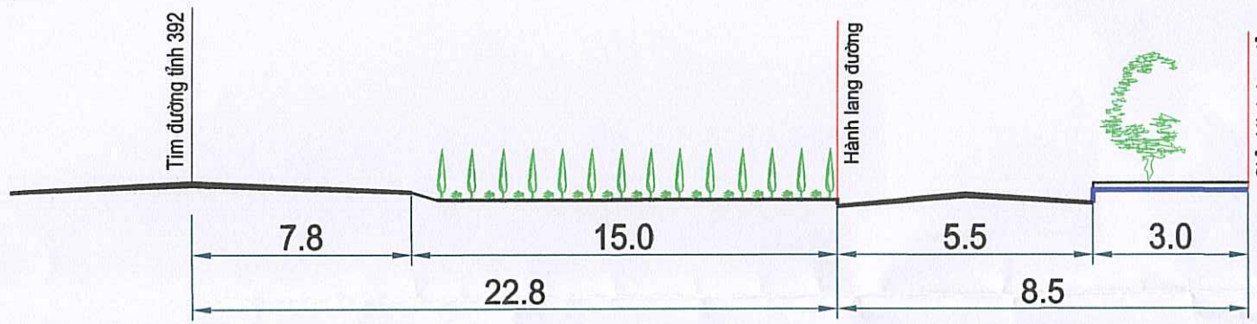
MẶT CẮT 1 - 1
