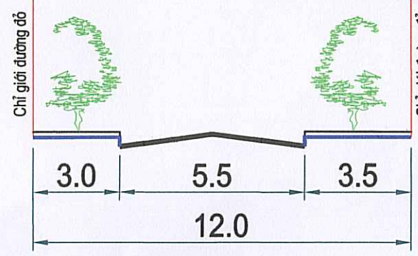
MẶT CẮT 4 - 4
