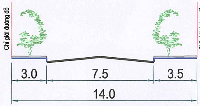
MẶT CẮT 3 - 3
