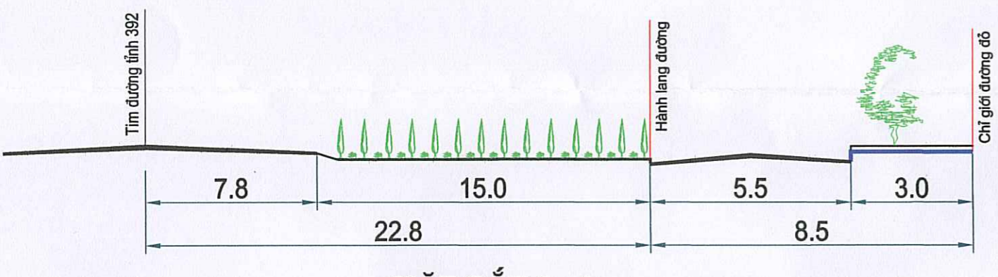
MẶT CẮT 1 - 1
