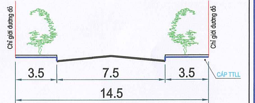
MẶT CẮT 2 - 2
