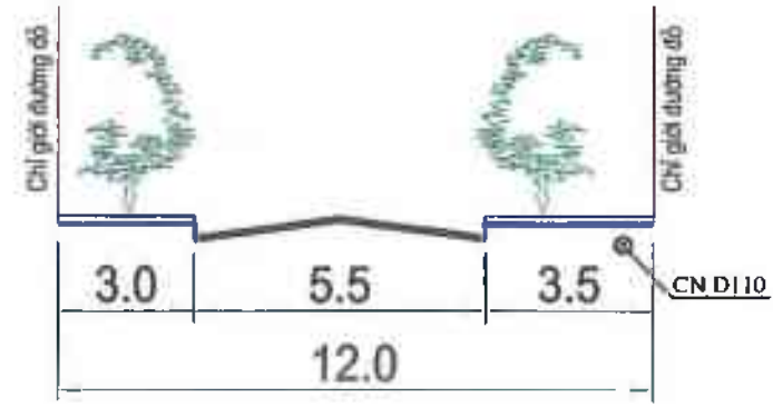
MẶT CẮT 4 - 4
