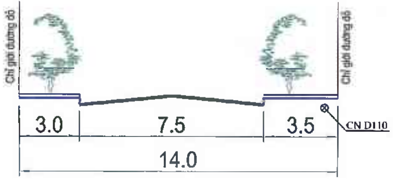
MẶT CẮT 3 - 3
