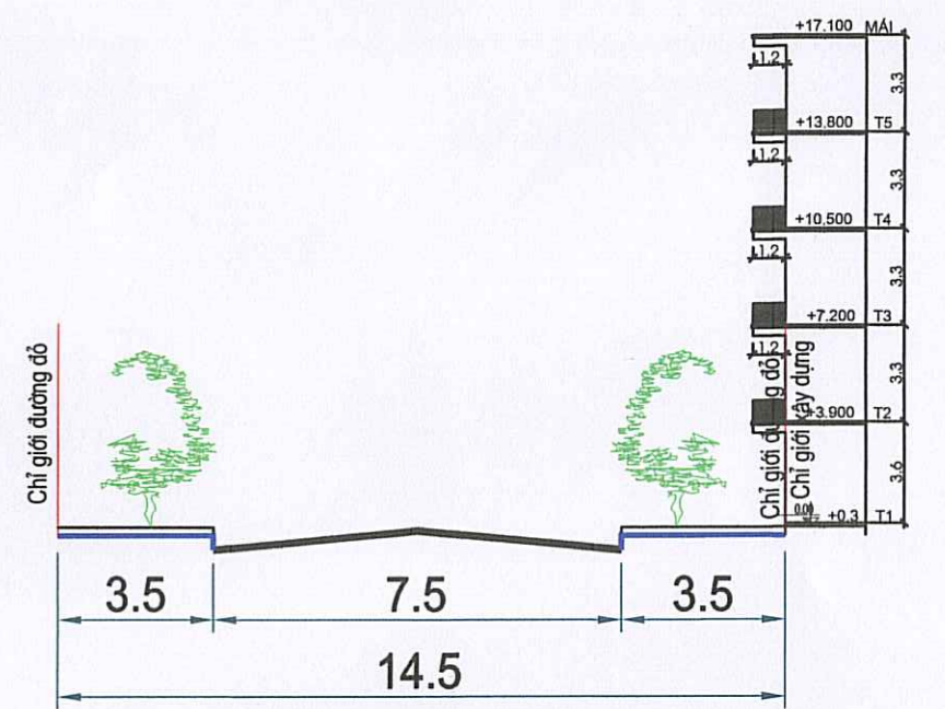
MẶT CẮT 2 - 2
