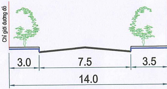
MẶT CẮT 3-3
