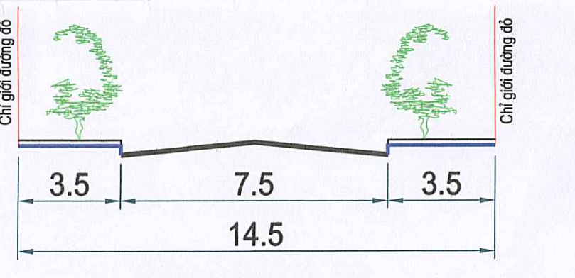
MẶT CẮT 2-2
