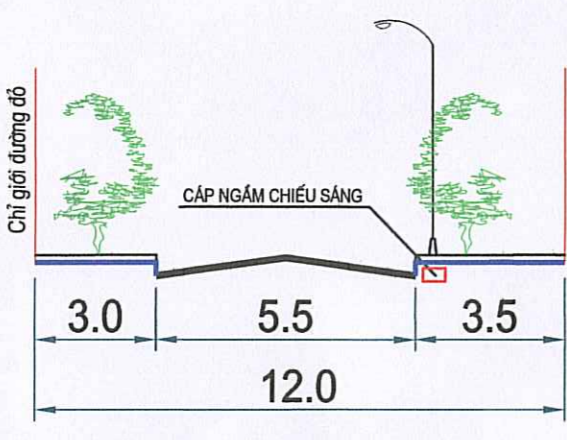
MẶT CẮT 4-4
