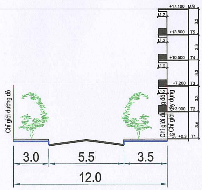
MẶT CẮT 4 - 4
