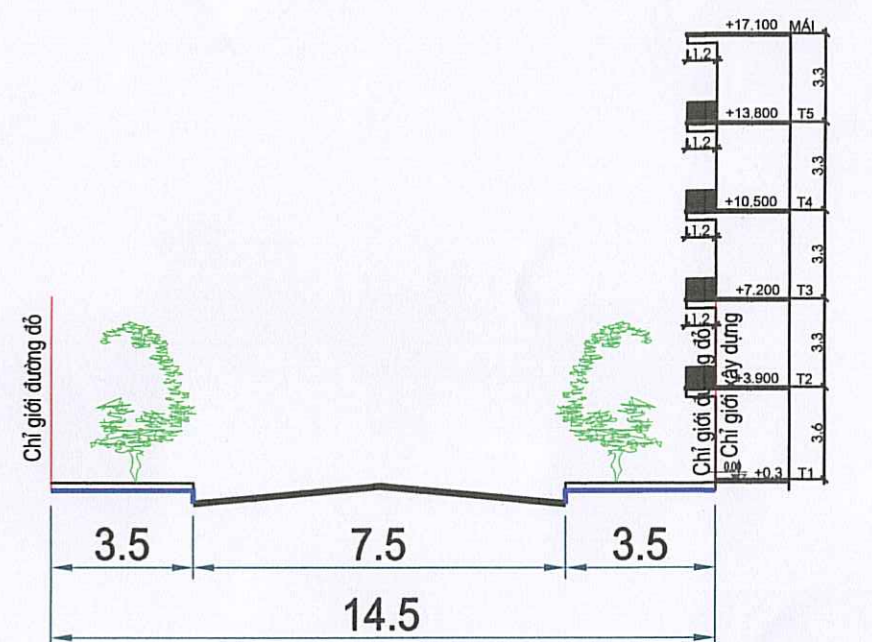
MẶT CẮT 2 - 2
