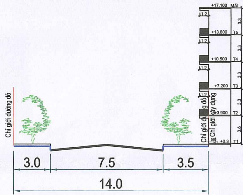
MẶT CẮT 3 - 3
