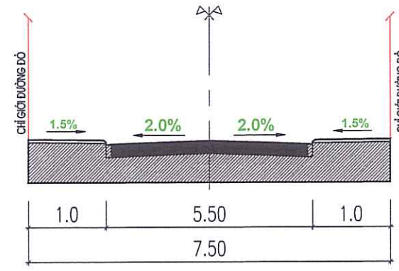
MẶT CẮT 1-1
