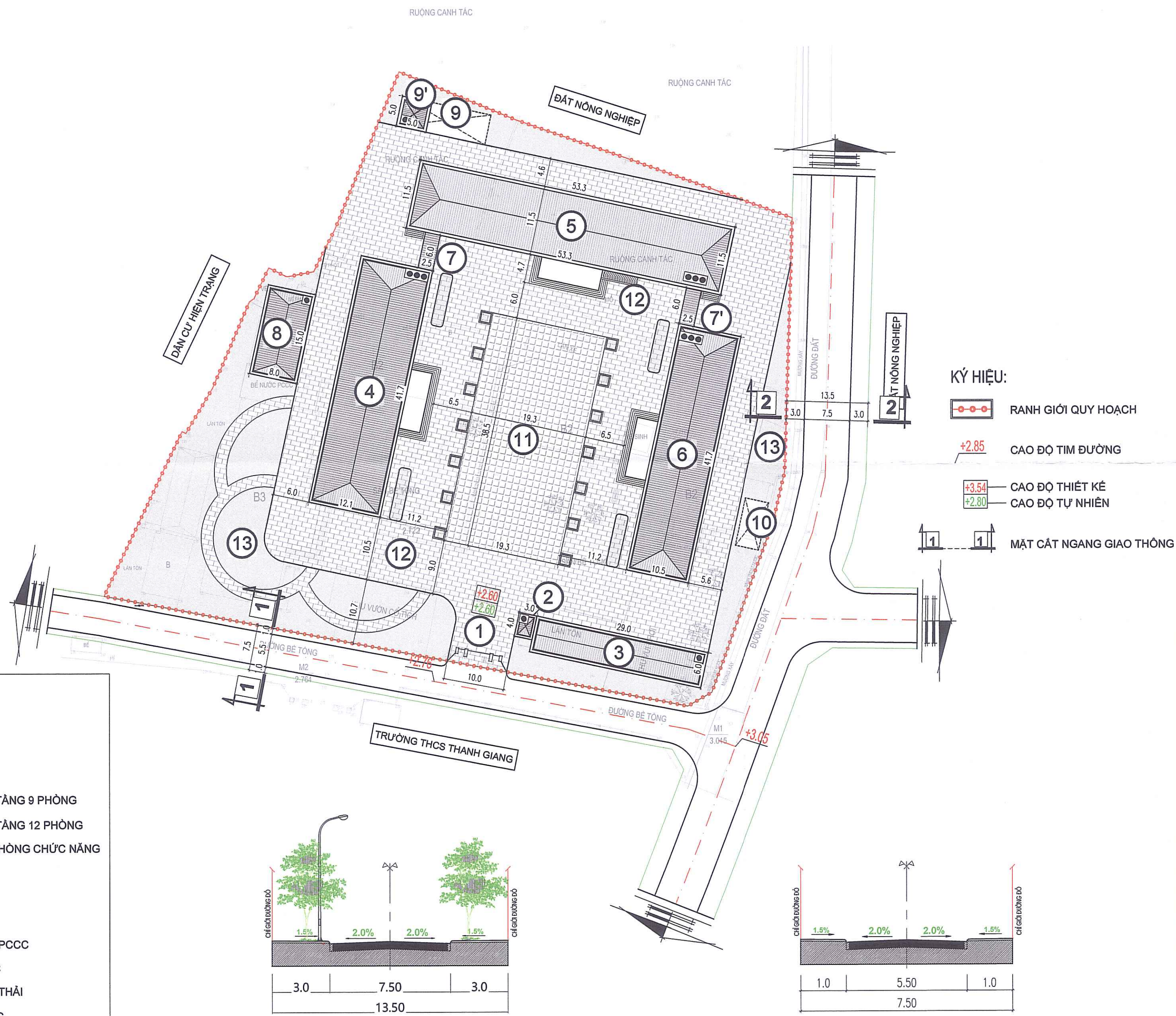
MẶT CẮT 2-2
