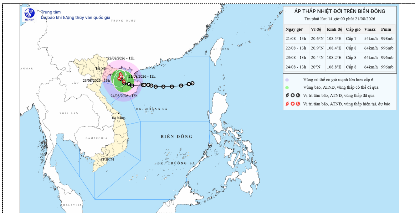
Hình 1. Bản đồ dự báo quỹ đạo và cường độ áp thấp nhiệt đới lúc 14h00 ngày 21/8/2026
