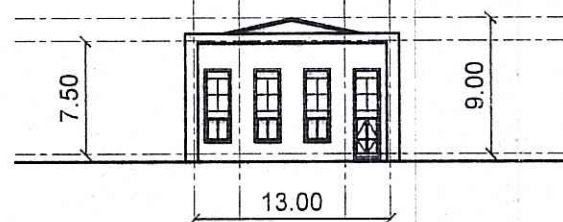
MẶT ĐỨNG 4
