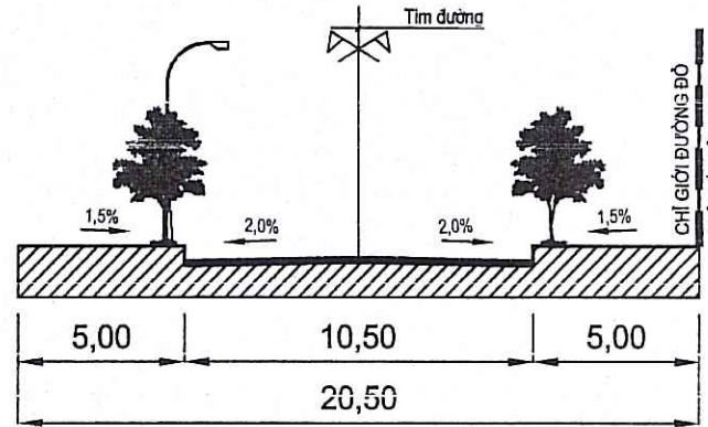
MẶT CẮT 1-1
