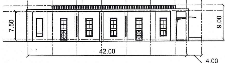
MẶT ĐỨNG 1
