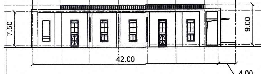
MẶT ĐỨNG 2
