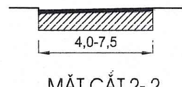
MẶT CẮT 2-2
