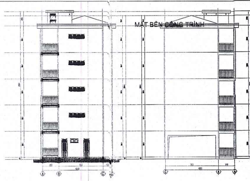
MINH HỌA MẶT ĐỪNG CÔNG TRÌNH
