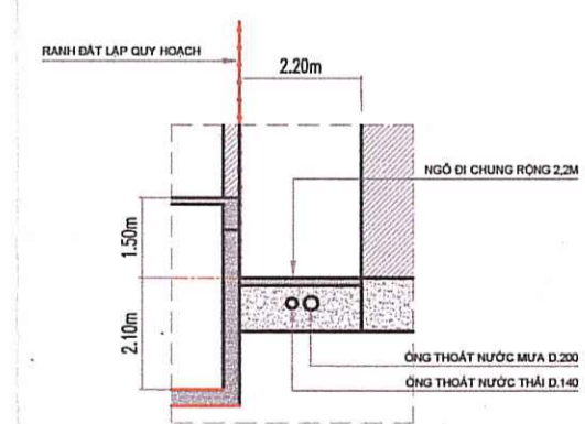
MẶT CẮT NGANG 2-2
