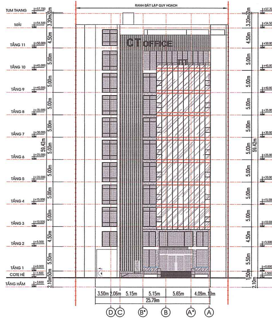
MẶT ĐỨNG TRỤC C-A
