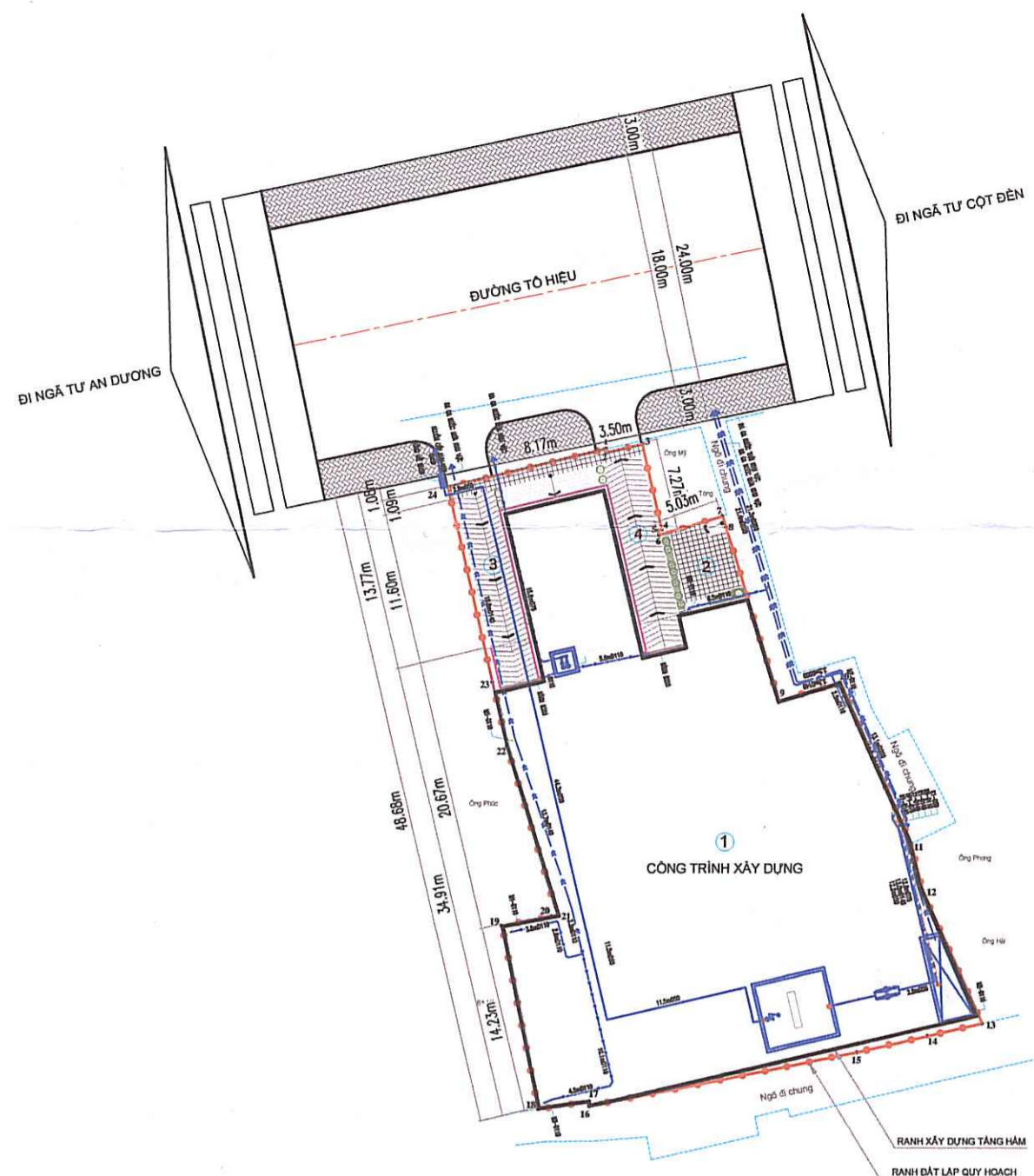
BẢN ĐỒ HỆ THỐNG CẤP THOÁT NƯỚC TỶ LỆ 1/500
