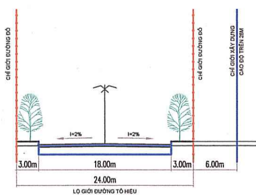
MẶT CẮT NGANG 1-1
