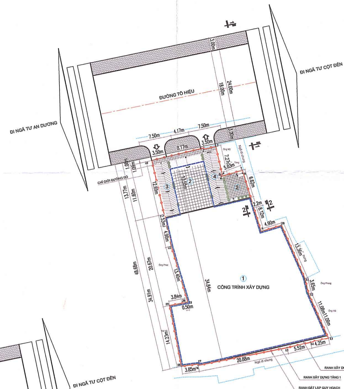
BẢN ĐỒ HỆ THỐNG GIAO THÔNG, CHỈ GIỚI ĐƯỜNG ĐỎ TỶ LỆ 1/500
