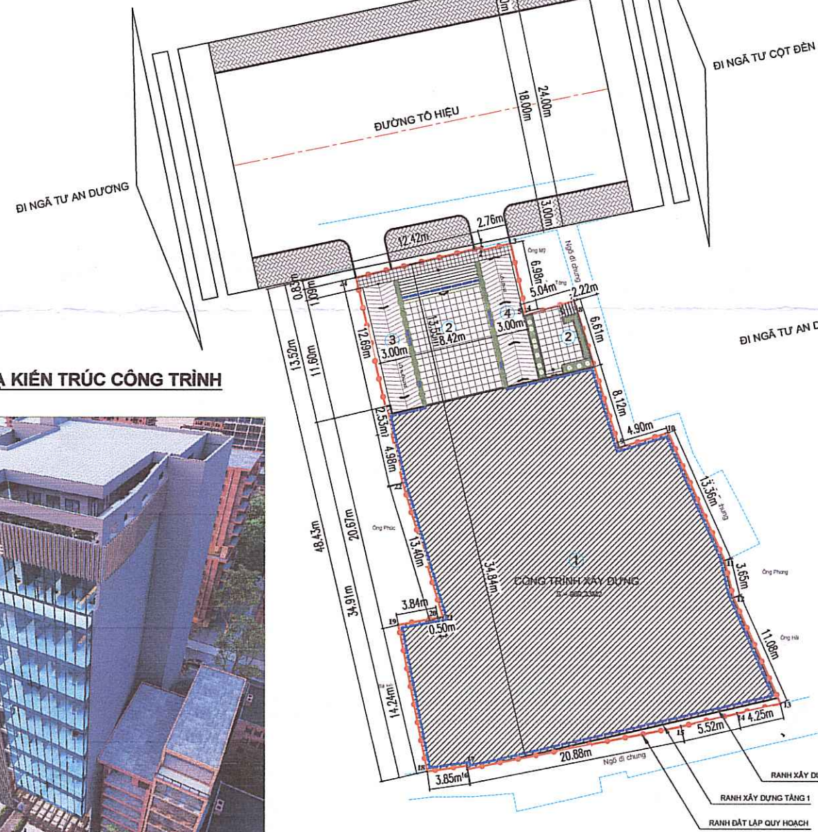
TỔNG MẶT BẰNG TẦNG 1 TỶ LỆ 1/500
