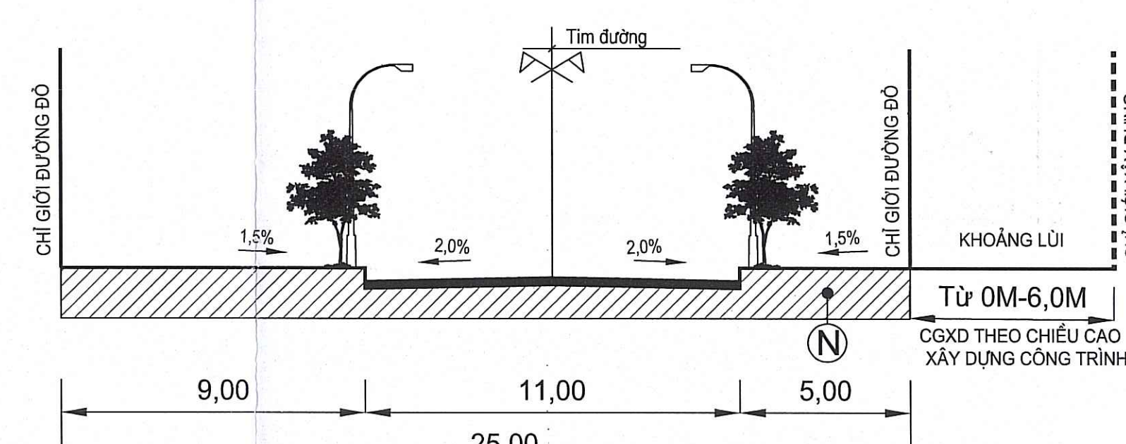
MẶT CẮT 1-1 (ĐƯỜNG NGUYỄN ĐỨC CẢNH)
