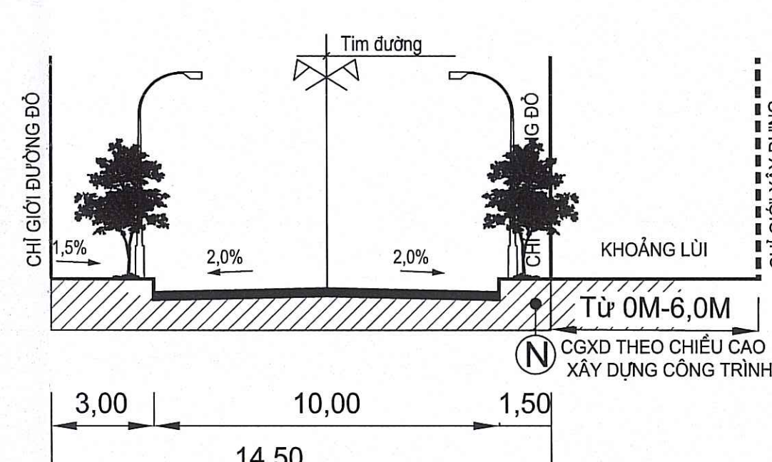
MẶT CẮT 2-2 (ĐƯỜNG NHÀ THƯƠNG)
