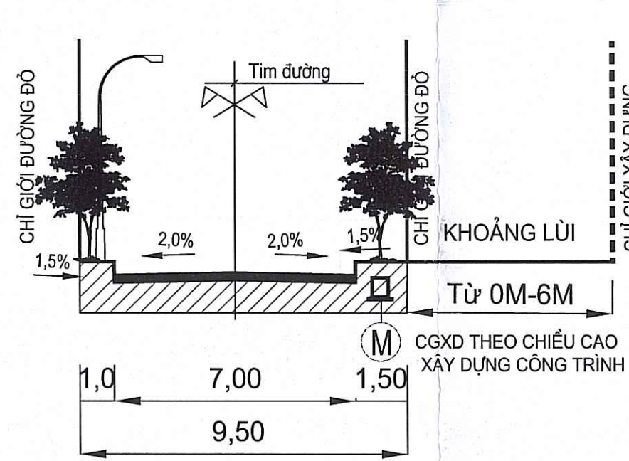
MẶT CẮT 2-2 (ĐƯỜNG NHÀ THƯƠNG)
