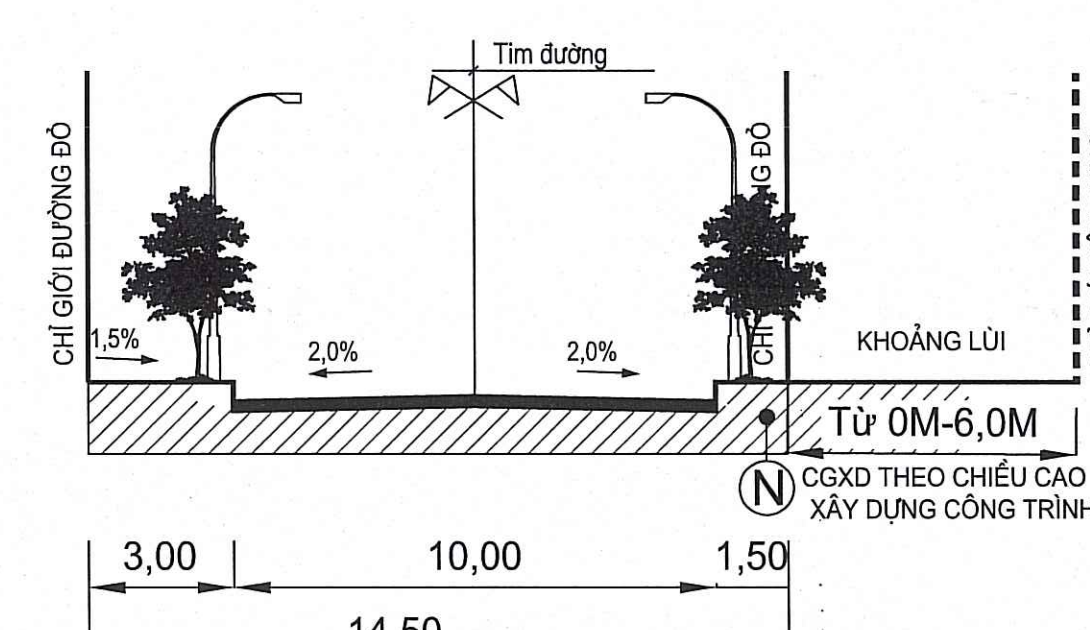
MẶT CẮT 2-2 (ĐƯỜNG NHÀ THƯƠNG)
