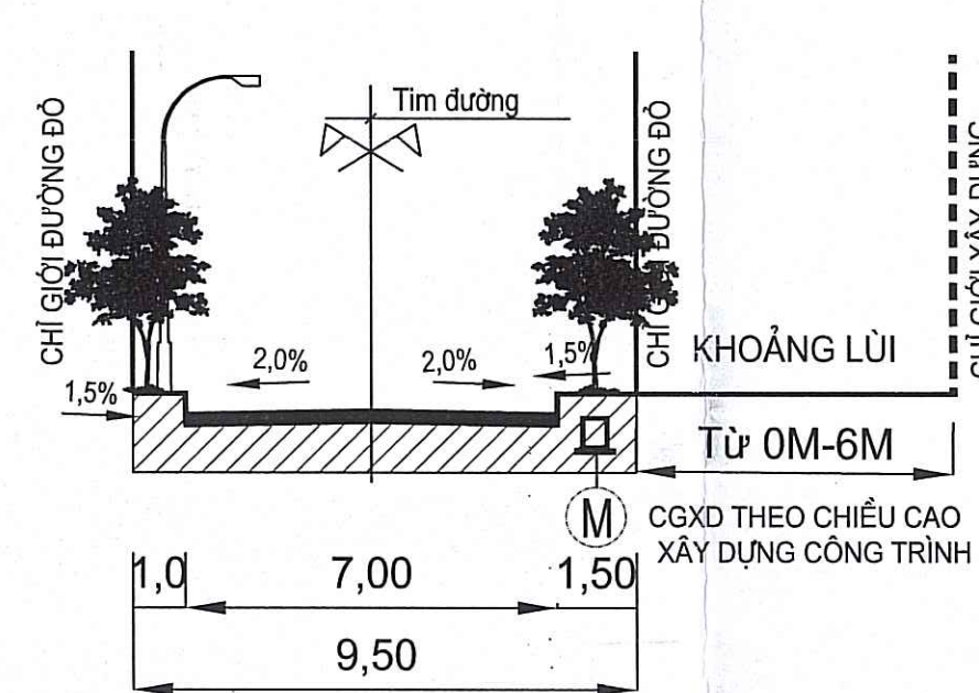
MẶT CẮT 2-2 (ĐƯỜNG NHÀ THƯƠNG)
