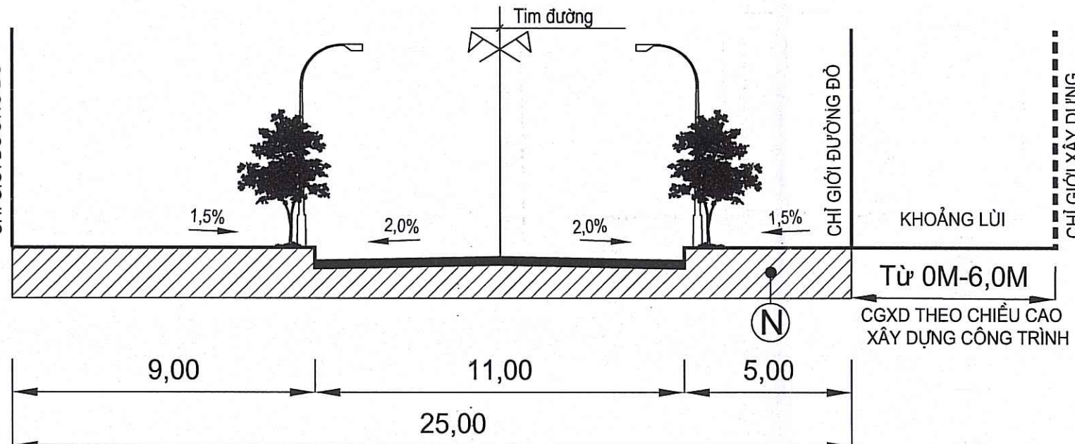
MẶT CẮT 1-1 (ĐƯỜNG NGUYỄN ĐỨC CẢNH)
