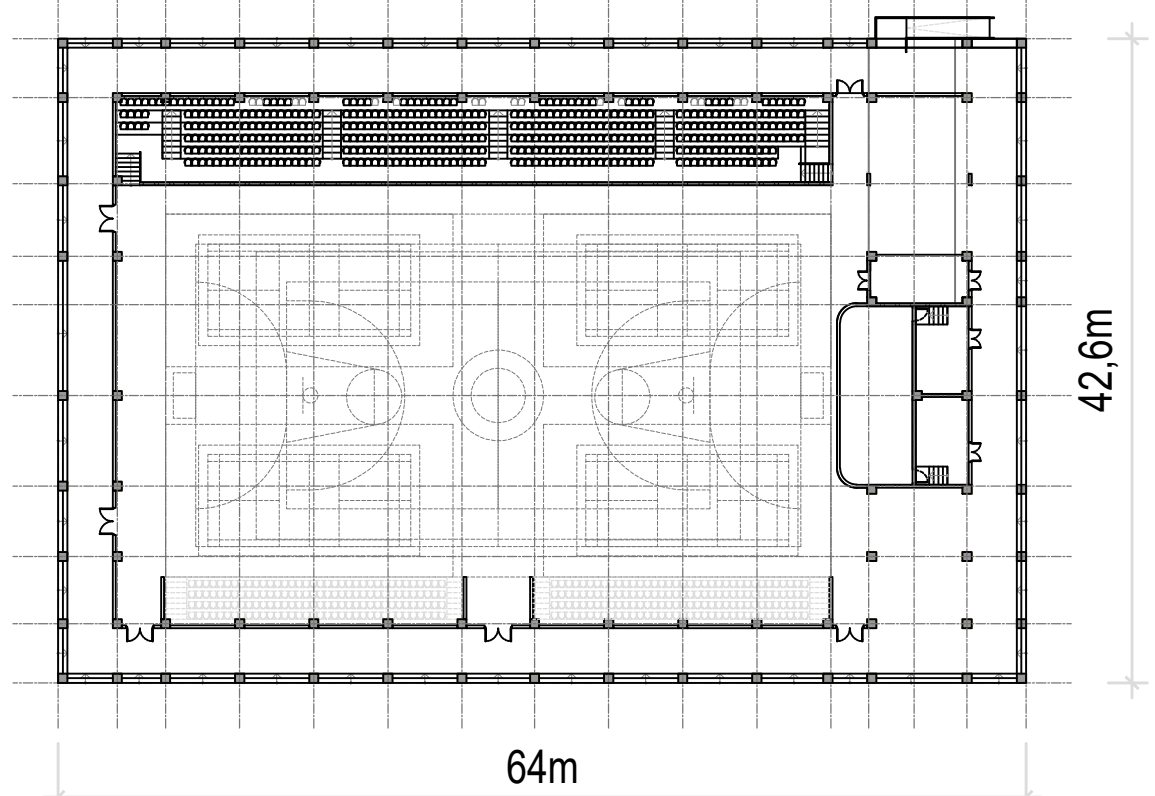
MB ĐIỂN HÌNH NHÀ ĐA NĂNG (09)
