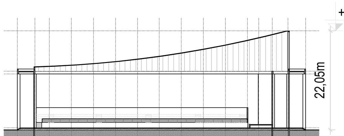
MẶT CẮT NHÀ ĐA NĂNG (09)
