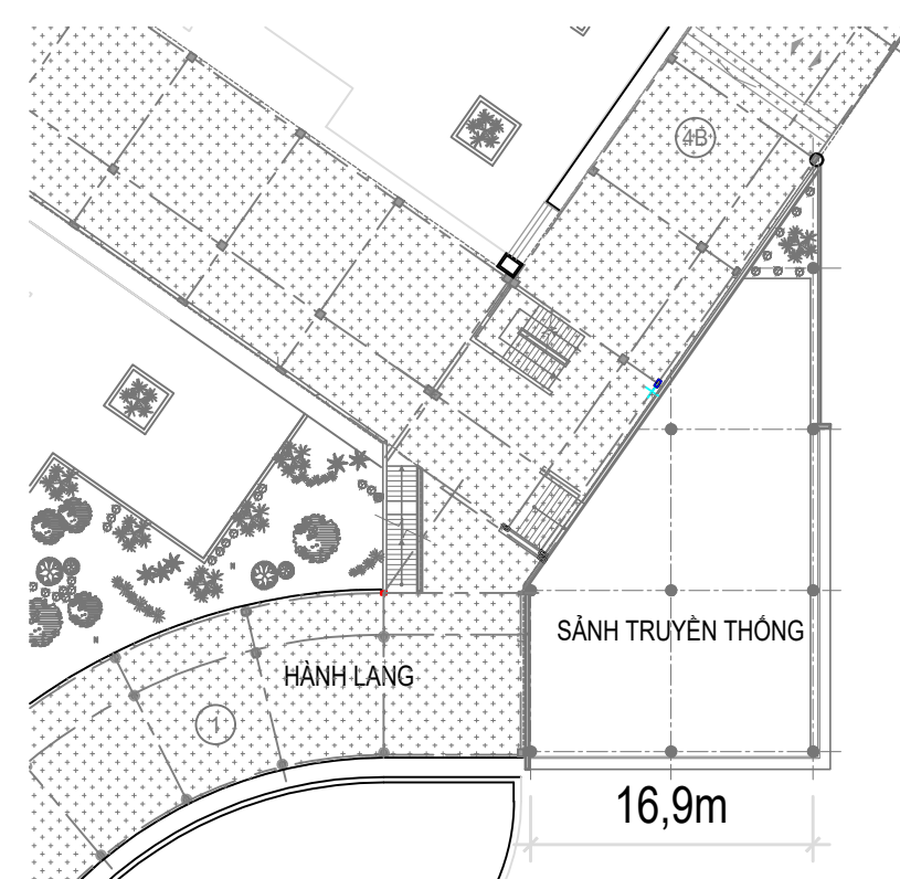
MB ĐIỂN HÌNH SÂN ĐÓN TIẾP (19)
