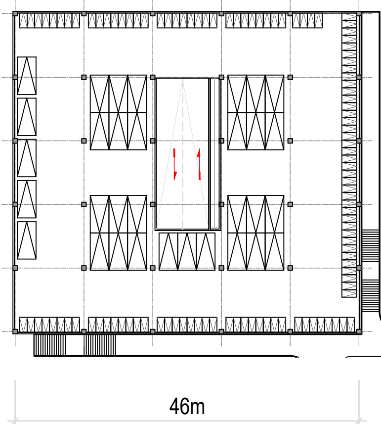
MB ĐIỂN HÌNH NHÀ ĐỂ XE HỌC SINH (07)
