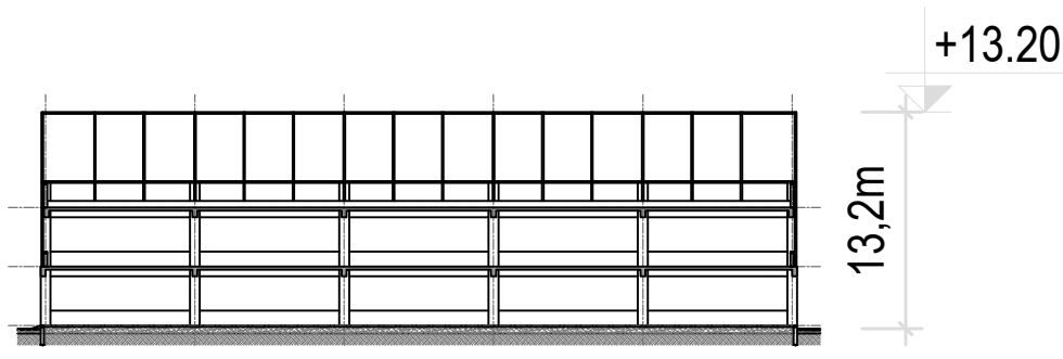
MẶT CẮT NHÀ ĐỂ XE HỌC SINH (07)
