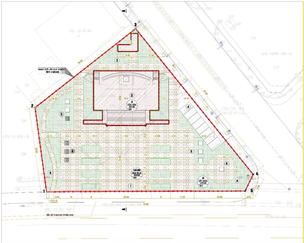
Mặt bằng tổng thể
