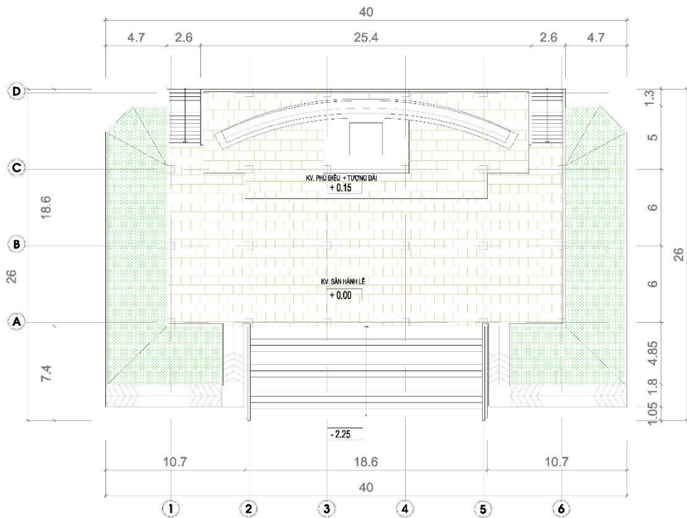
MẶT BẰNG CỘT +0.00
