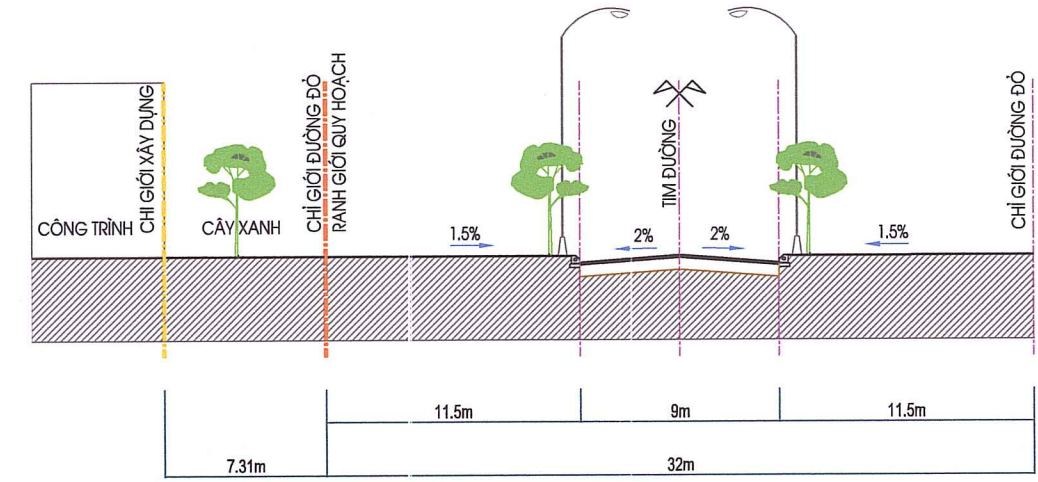
MẶT CẮT 1-1
