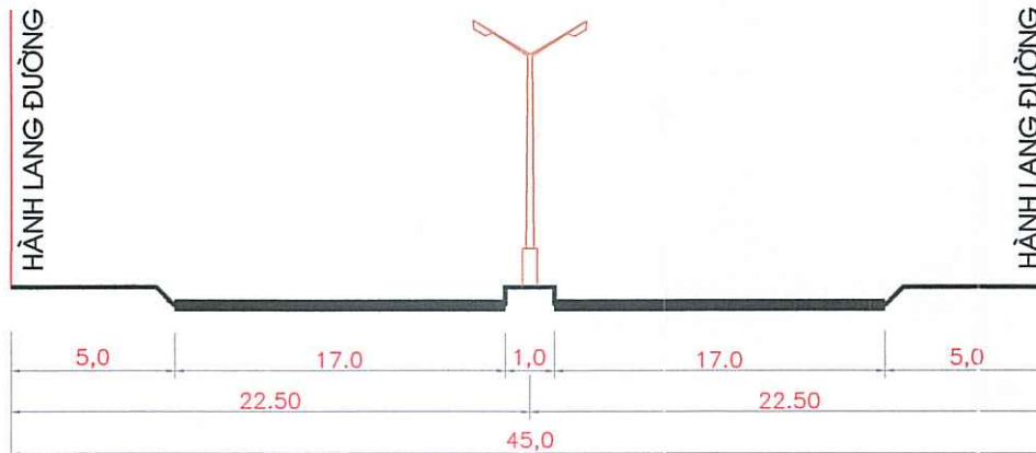
MẶT CẮT 1-1
