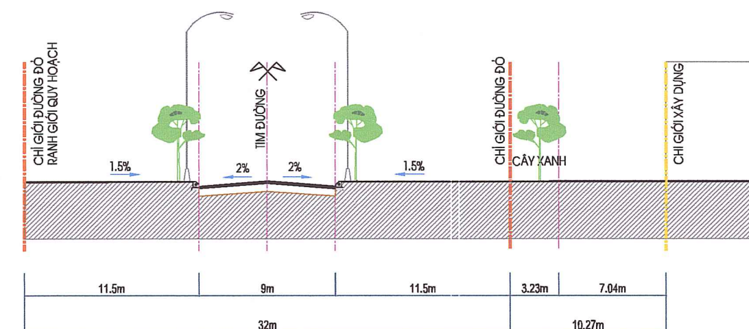
MẶT CẮT 1-1
