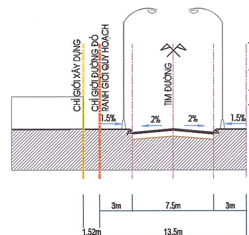
MẶT CẮT 2-2
