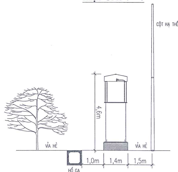
MẶT CẮT 1 - 1
