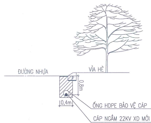
MẶT CẮT 3 - 3
