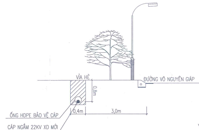
MẶT CẮT 4 - 4
