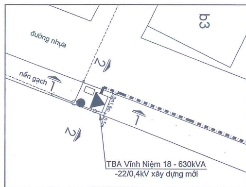
TRÍCH A (MẶT BẰNG VỊ TRÍ TBA VĨNH NIỆM 18)
