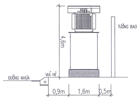
MẶT CẮT 2 - 2
