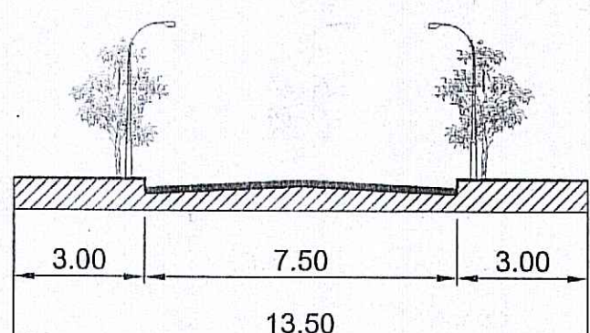
MẶT CẮT 3-3
