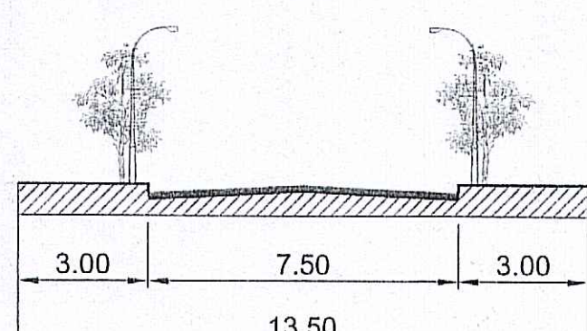
MẶT CẮT 4-4
