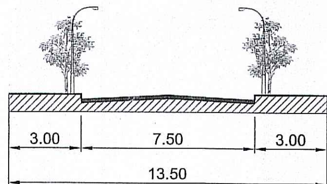
MẶT CẮT 2-2
