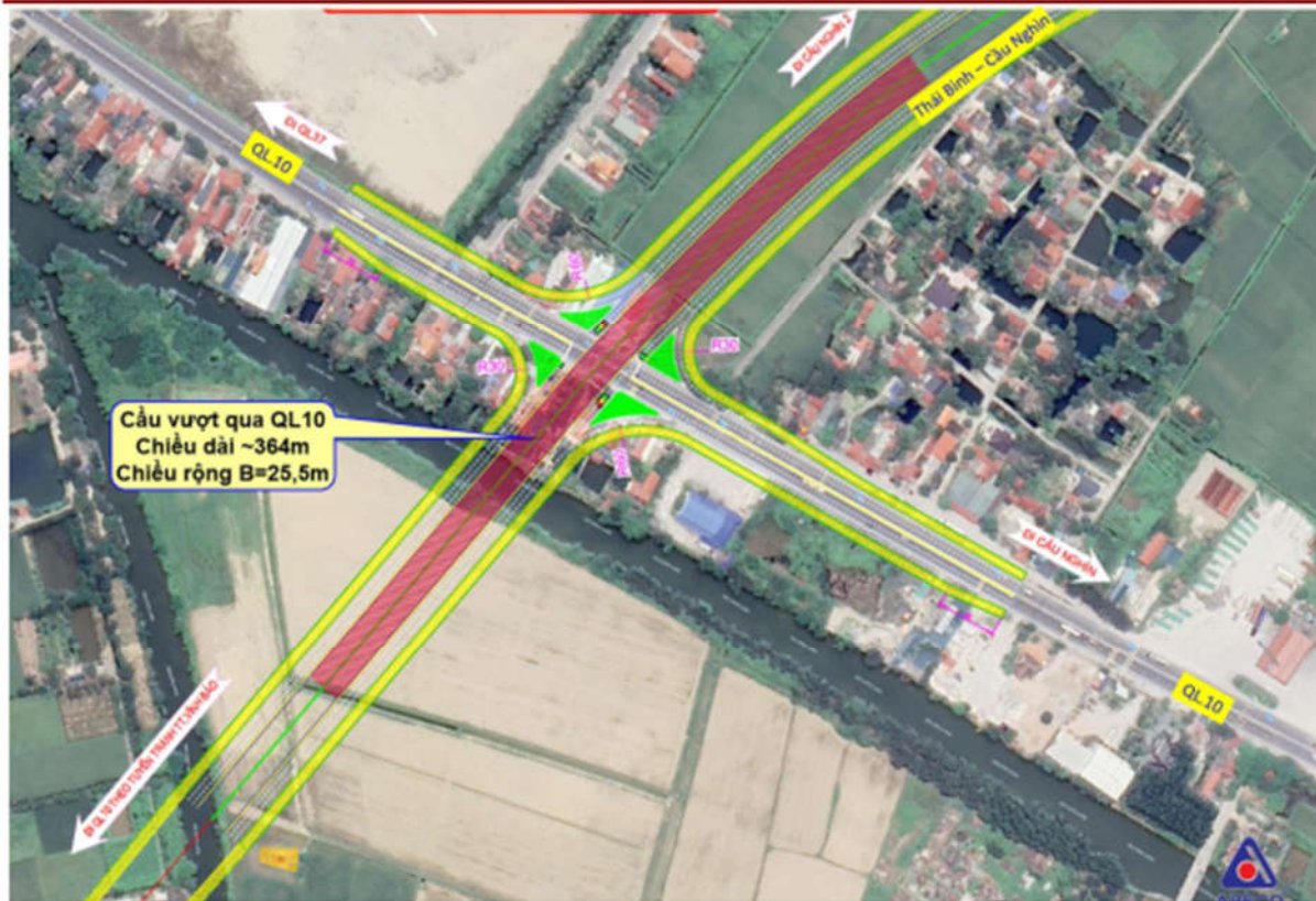
(Mặt bằng nút giao cuối tuyến với Quốc lộ 10)
