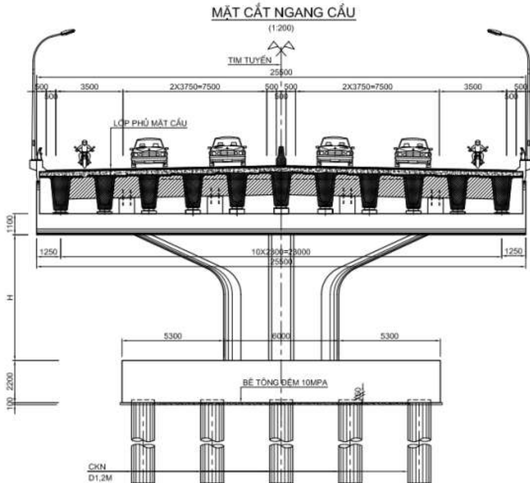
(Mặt cắt ngang cầu vượt Quốc lộ 10 – phương án 2)
