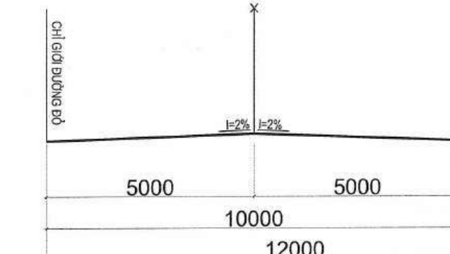
MẶT CẮT 5-5
