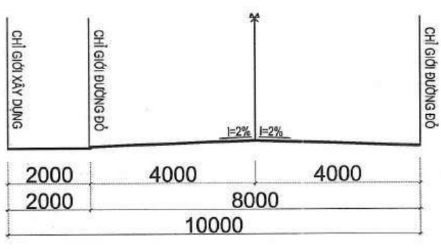
MẶT CẮT 1-1
