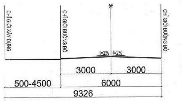
MẶT CẮT 2-2
