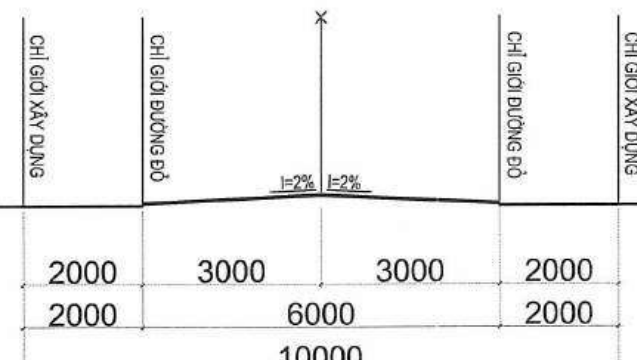
MẶT CẮT 4-4
