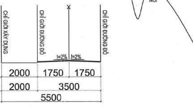
MẶT CẮT 3-3
