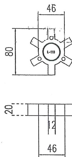
GIẢM CHẤN CAO SU
