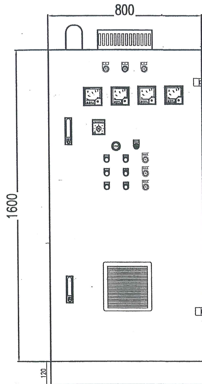
MẶT TRƯỚC
