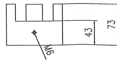
CHI TIẾT 3
