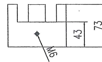
CHI TIẾT 4
