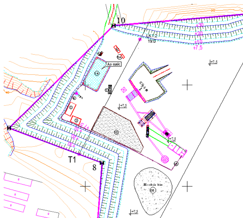
Hình 4. Sơ đồ bố trí công trình xử lý nước thải công nghiệp (số 6, 6A là bể xử lý nước rửa xe có bể tách dầu)
